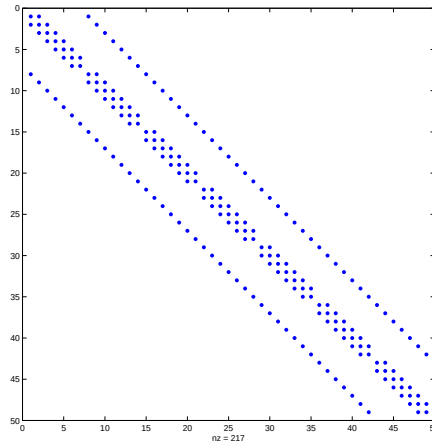
Slika 2.1: Uzorak popunjenosti matrice A koja se pojavljuje u diskretizaciji Poissonove jednadžbe s 5-točkovnim operatorom na 7 \times 7 mreži.
