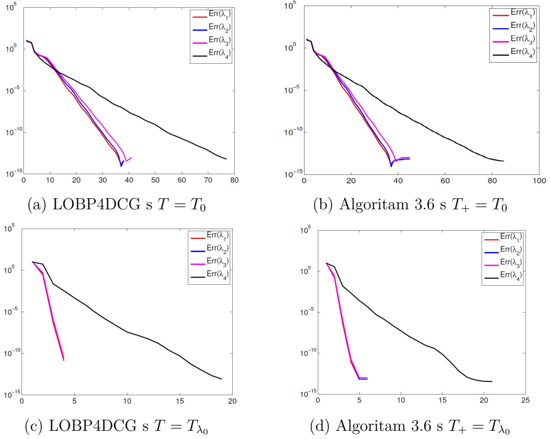
Slika 3.2: Relativne pogreške izračunatih pozitivnih svojstvenih vrijednosti primjenom LOBP4DCG-a i Algoritma 3.6 na matričnom paru iz Eksp. 3.12.
