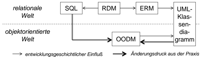
Abbildung 1: Beziehung der in dieser Arbeit herangezogenen Modelle und deren Notationen. Wir leiten aus dem Änderungsdruck unter Berücksichtigung der Entwicklungsgeschichte eine sanfte Erweiterung des OODMs um relationale Aspekte ab.
