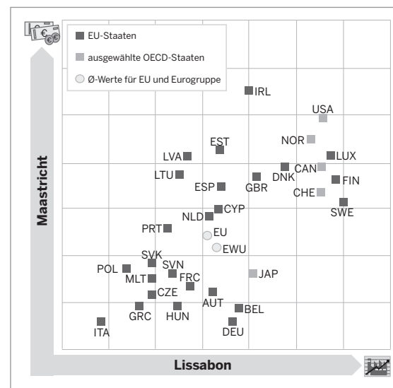
Abbildung 1: Der LiMa-Benchmark,
