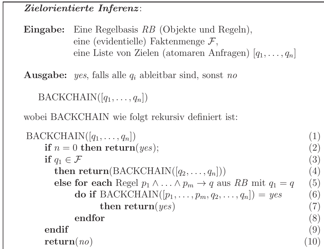
Abbildung 4.5: Algorithmus zur zielorientierten Inferenz
